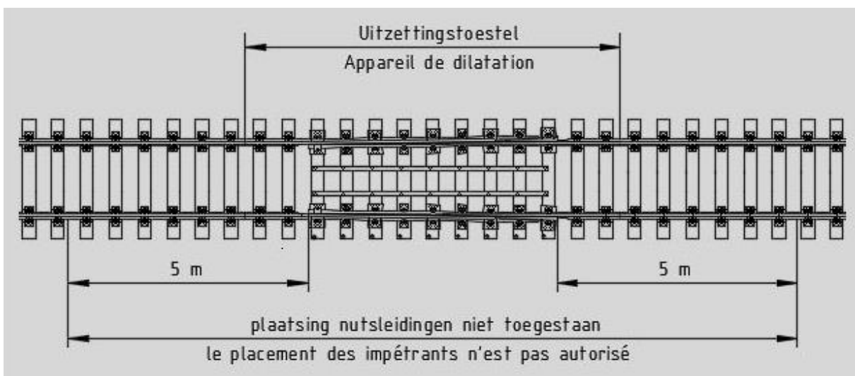
Figure 2.3 : zone à risque pour la pose d'impétrants dans le cas d'un appareil de dilatation
