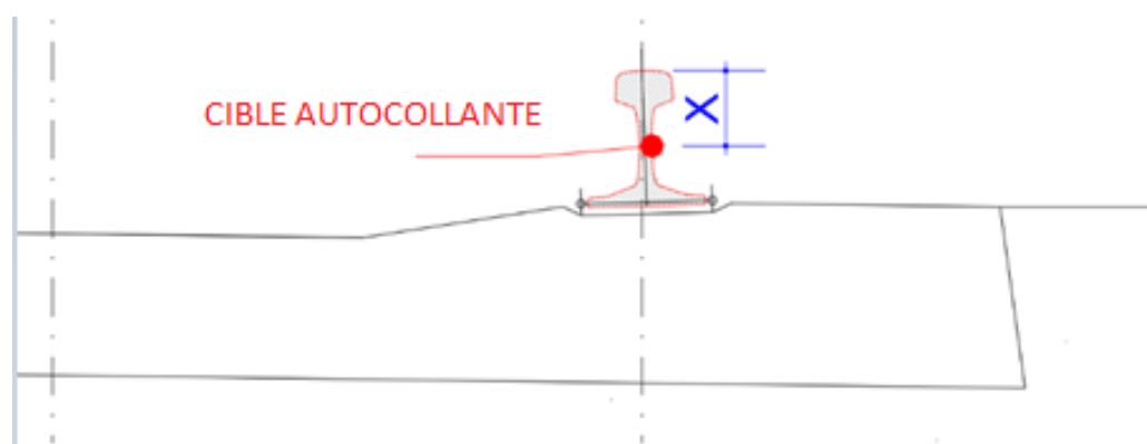
Figure 2.10 : Placement de cible
