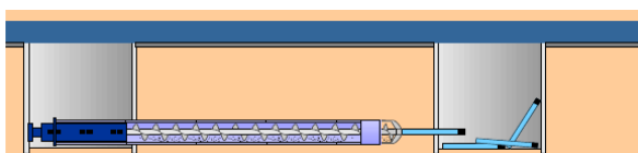
Figure 2.18 : Fonçage avec tige pilote –curage à la tarière
