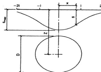
Figure 2.20 : caractéristiques de la courbe de probabilité dans le cas d'une cuvette de tassement au-dessus d'un tunnel circulaire
