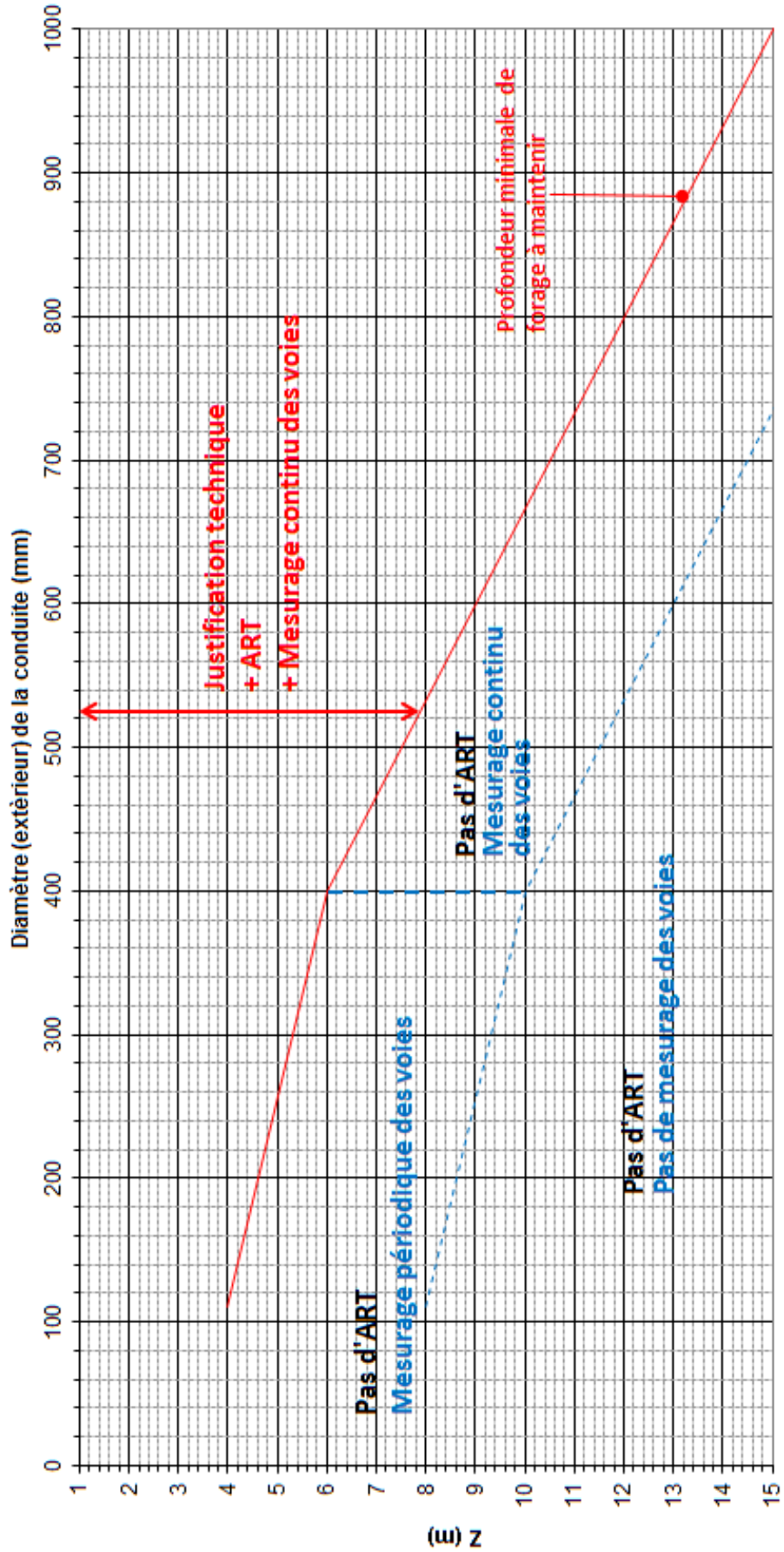
Figure 2.26 : Profondeur de forage minimale à respecter
