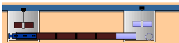
Figure 2.19 : Fonçage avec tige pilote –post-fonçage de la conduite
