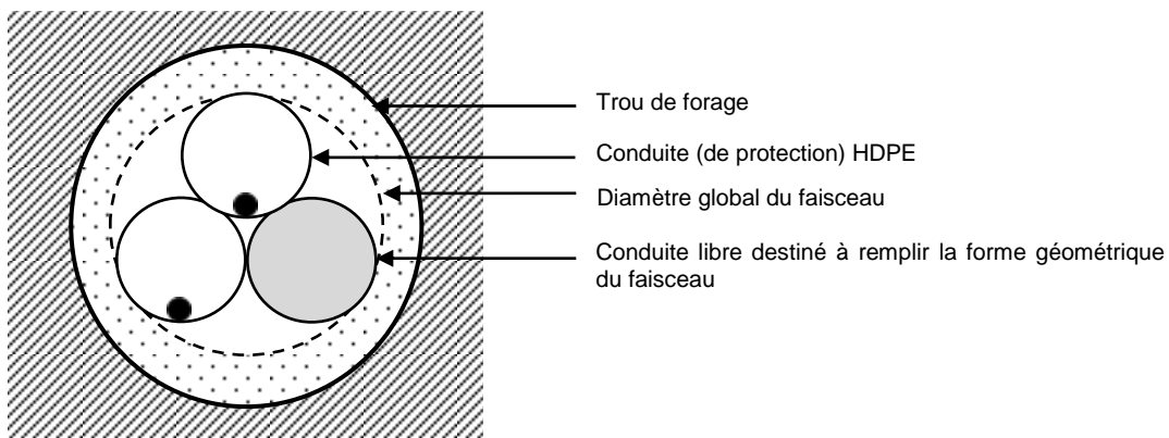
Figure 2.5 : Coupe transversale du trou de forage
