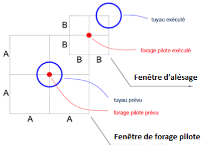
Figure 2.25 : Tolérances fenêtre pilote-alésage
