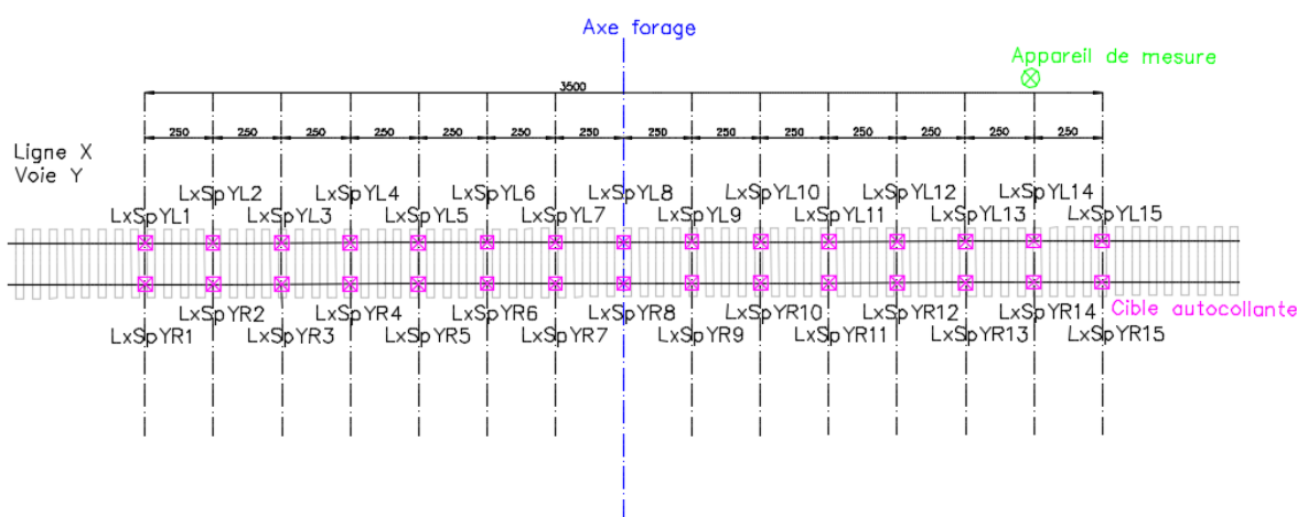
Figure 2.9 : Zone de travail - vue en plan
