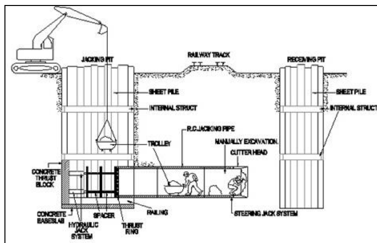
Figure 2.13 : Technique du front ouvert
