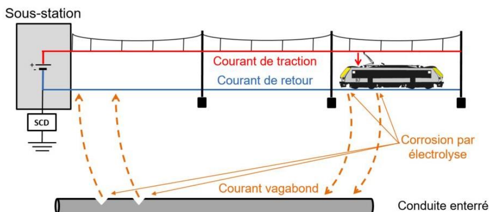
Figure 2.27 : Courants vagabonds et corrosion électrolytique
