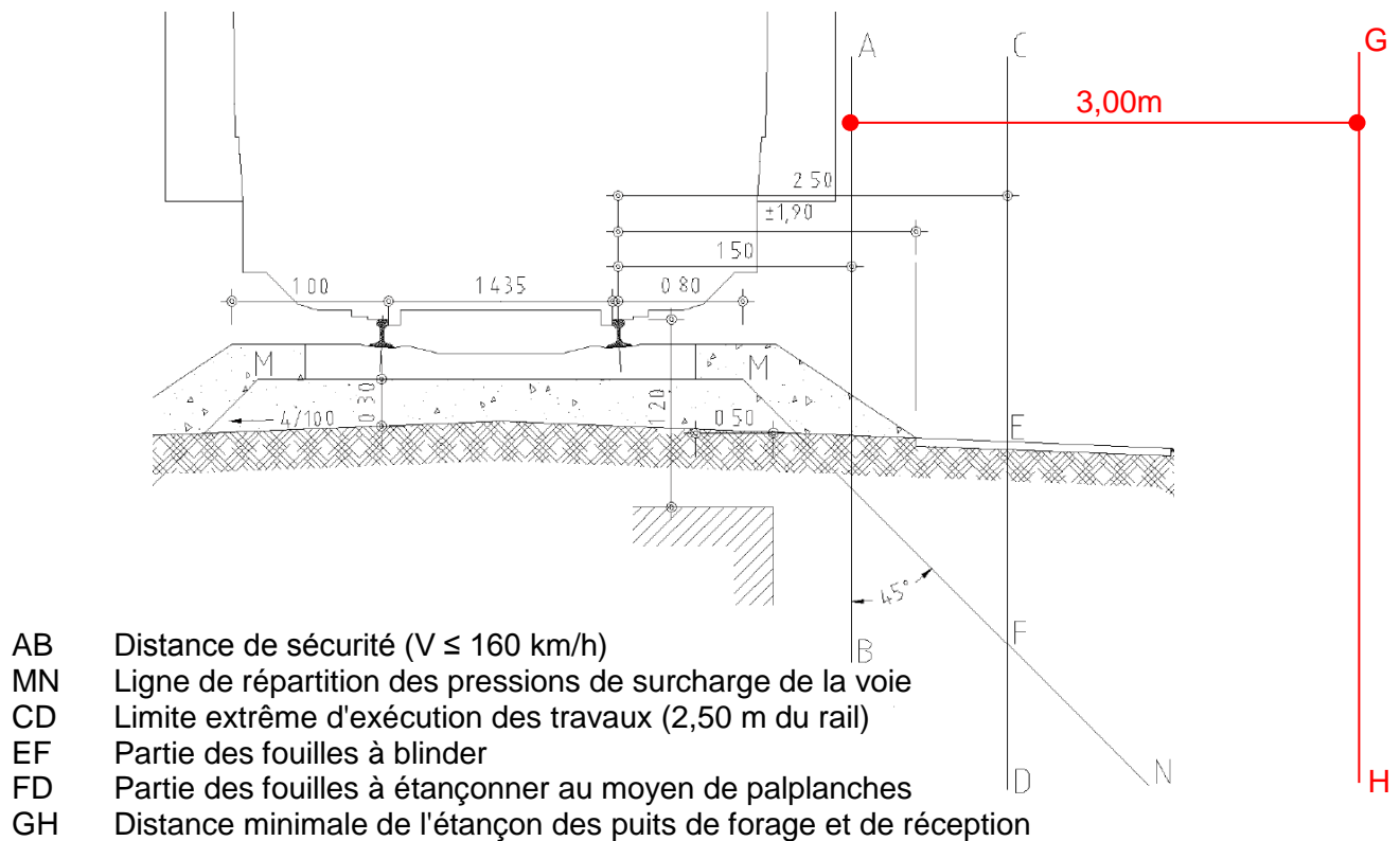
Figure 2.11 : Fouilles à côté des voies
